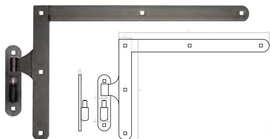
Zawias kątowy Hinge / Петля / Scharnier
