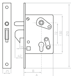
Zamek hakowy Lock / Врезной замок / Hackenschloss
