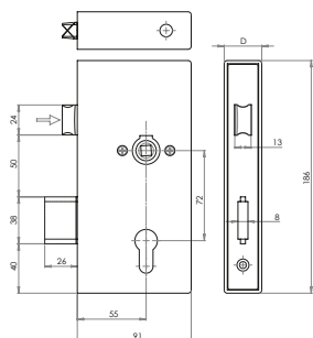
Kaseta z zamkiem Lock box set / Врезной замок + корпус замка / Schloss + Kasten
