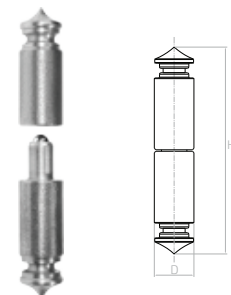
Zawias ozdobny z kulą Welding hinge with ball / Петля приварная с шаром / Scharnier mit Kugel
