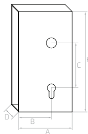
Obudowa zamka Lock box / Корпус замка / Schlosskasten
