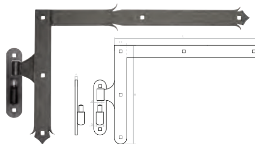
Zawias kątowy ozdobny Hinge / Петля / Scharnier
